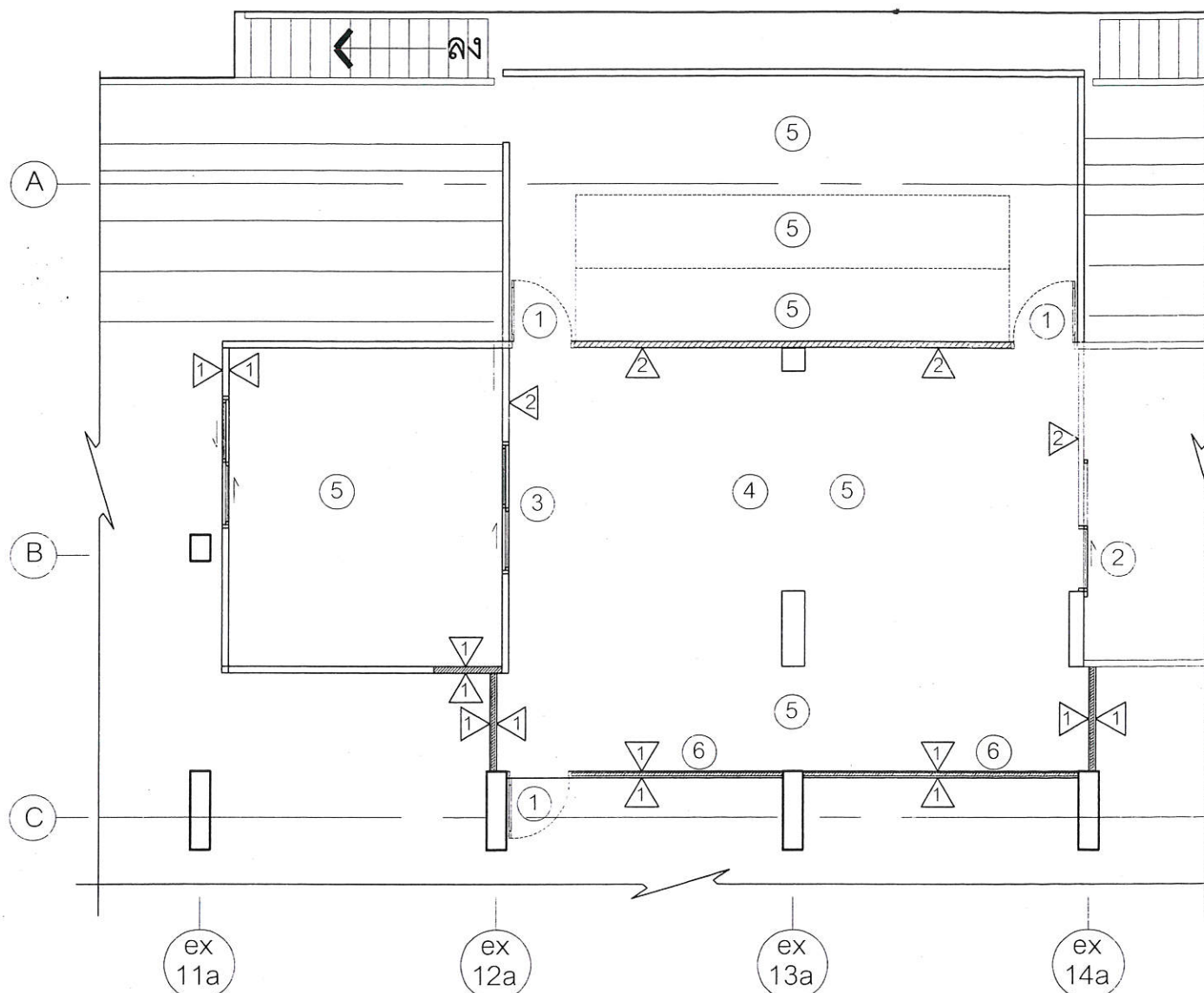
แปลนปรับปรุงห้องรับรองชั้น 2 อาคารสนามกีฬากลาง SCALE 1:100
